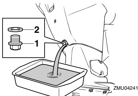
1. Tornillo de drenaje 2. Junta
