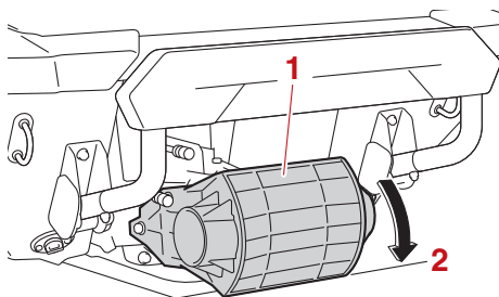
1 Compuerta de inversión 2 Posición de marcha atrás
