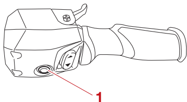
1 Interruptor de arranque/paro del motor
